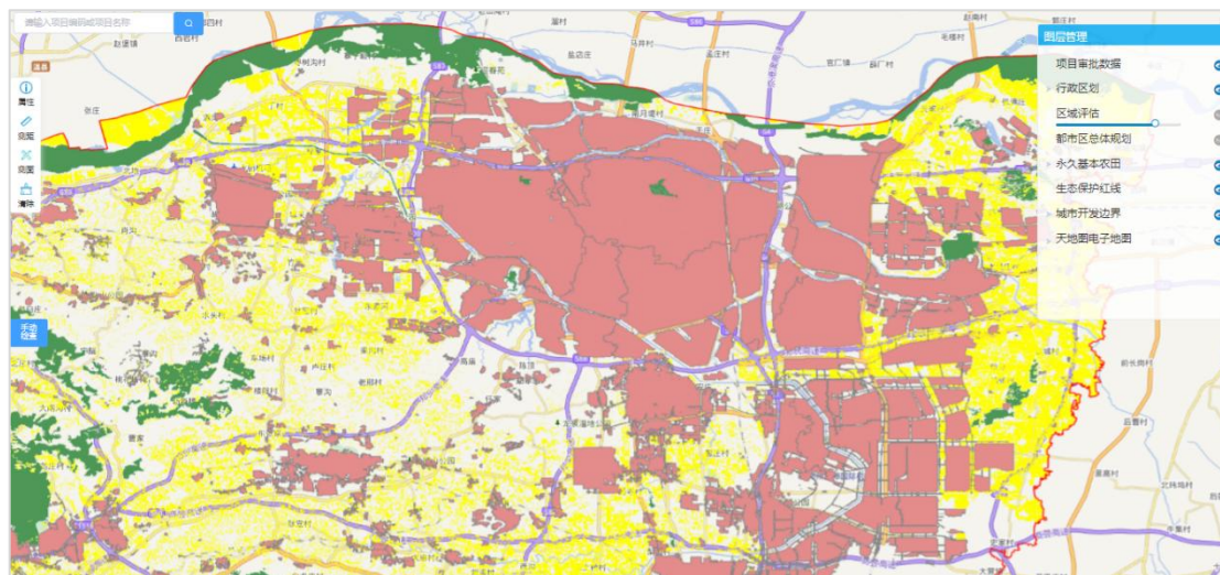
图 7-1 省共享页面
