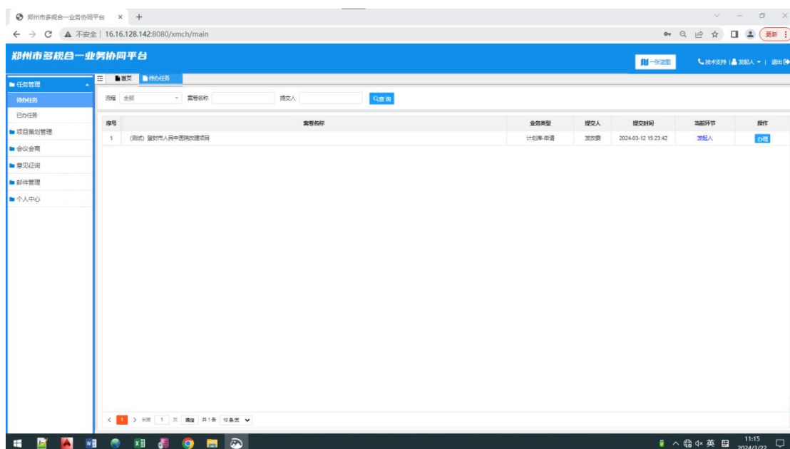
图 3-3 待办任务
