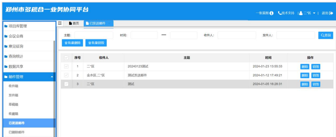
图 5-5 已发送邮件
