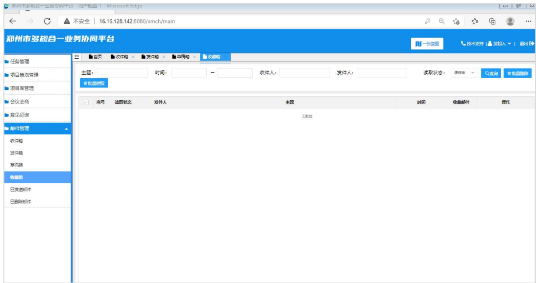
图 5-4 收藏箱
