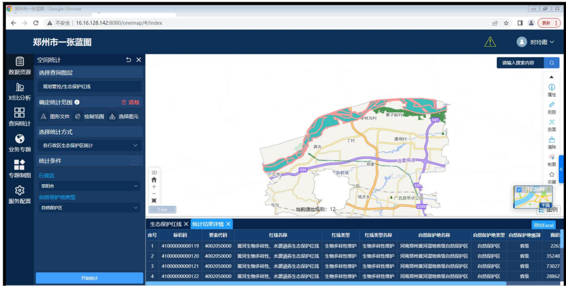
图 8-4 空间统计
