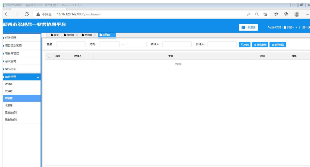
图 5-3 草稿箱
