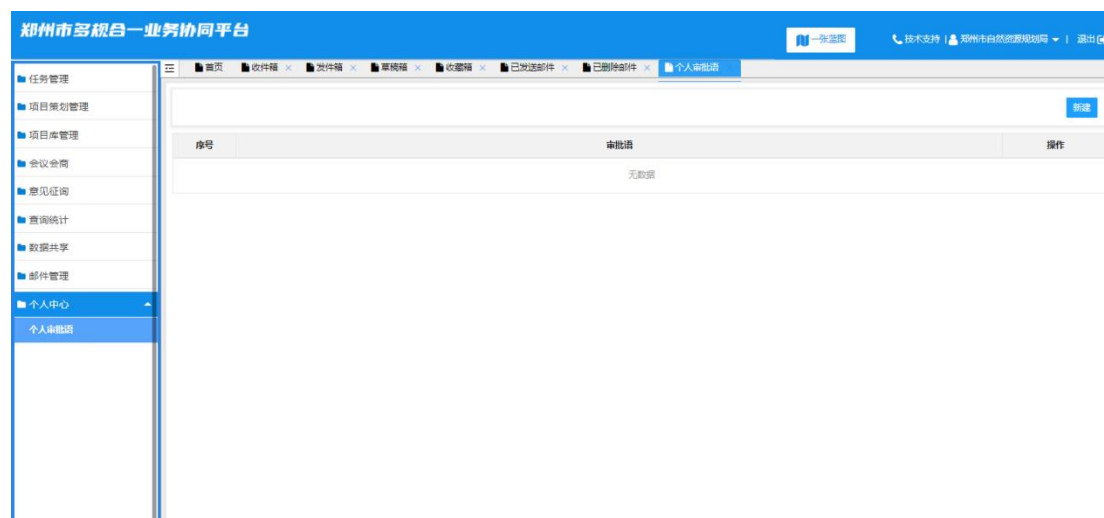
图 6-11 个人审批语
